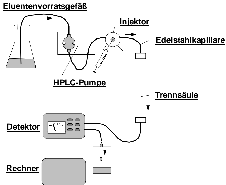
1 Schema eines HPLC - Systems
