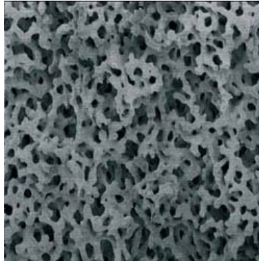
1 Monolithisches Kieselgel (Quelle: Merck Chrombook 2004)
