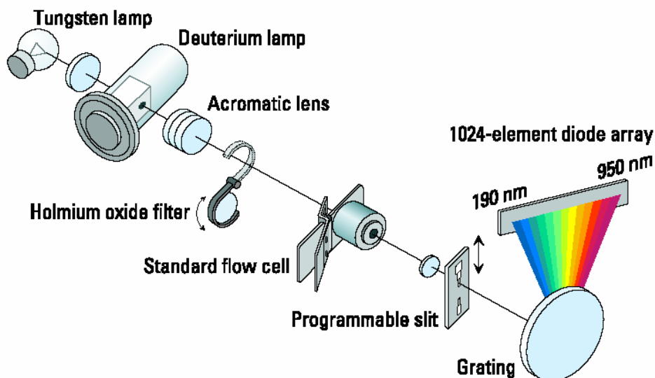
1 Prinzip eines HPLC-UV-Detektors mit variabler Wellenlänge
