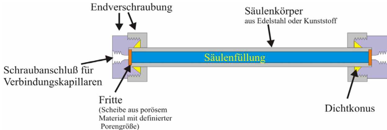
1 Aufbau einer HPLC - Trennsäule
