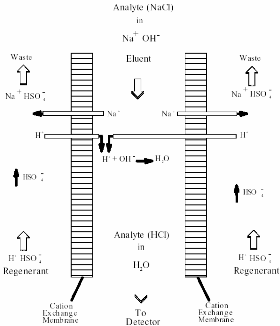
1 Funktionsschema eines Membransuppressors für die Anionenchromatographie (Quelle: Dionex – Handbuch für AMMS III)
