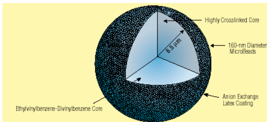
1 Partikel für Anionentrennsäulen (Quelle: Dionex – Prospekt für Säule AS4A-SC)
