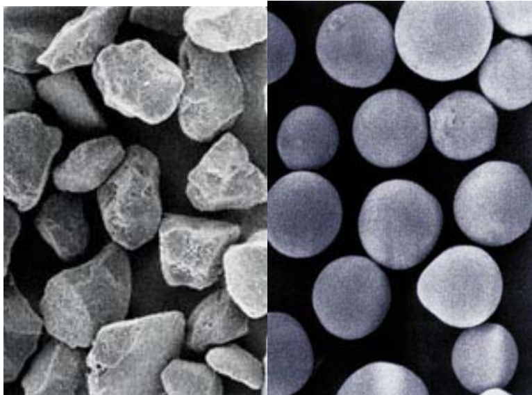
1 REM - Aufnahmen von irregulärem und sphärischem Kieselgel (Quelle: Merck Chrombook 2004)
