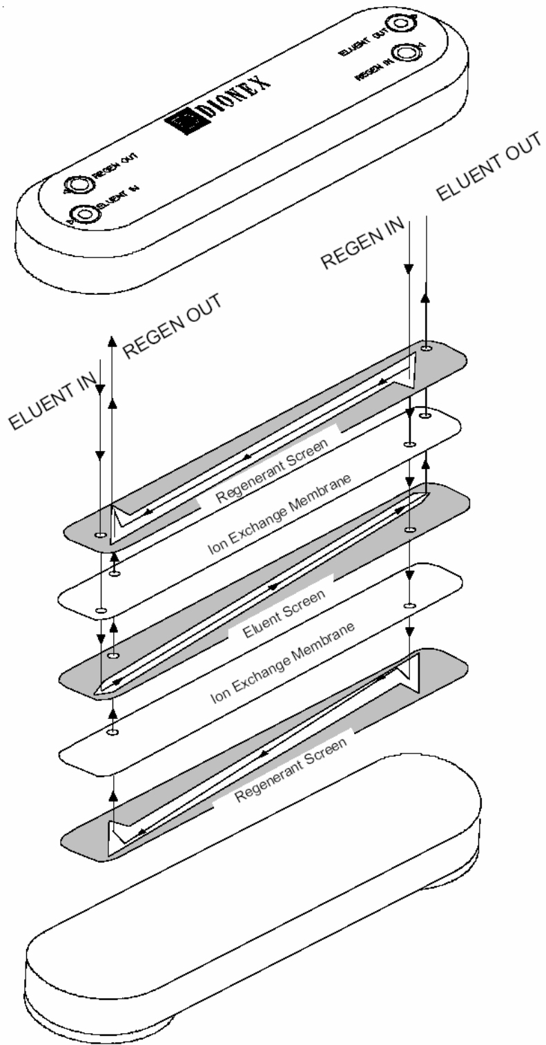
1 Explosionszeichnung eines Membransuppressor (Quelle: Dionex – Handbuch für AMMS III)
