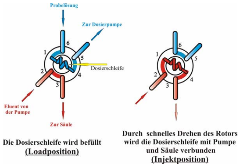
1 Funktionsschema eines HPLC-Injektionsventils
